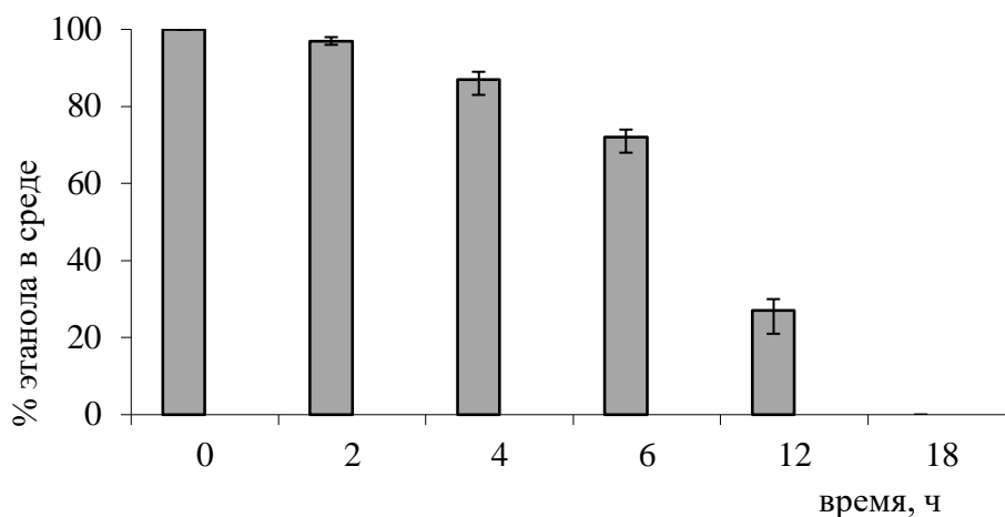
Рис. 1. Биодegradация ксенобиотика бактериями L. gasseri БИМ В-1912
